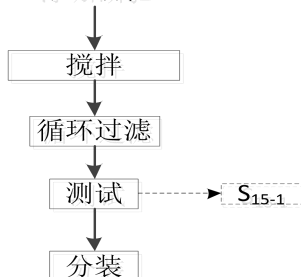
图 12 RDT500 248nm 厚膜光刻胶项目工艺流程图
