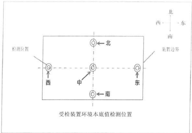
环境浓度及气象信息采集
